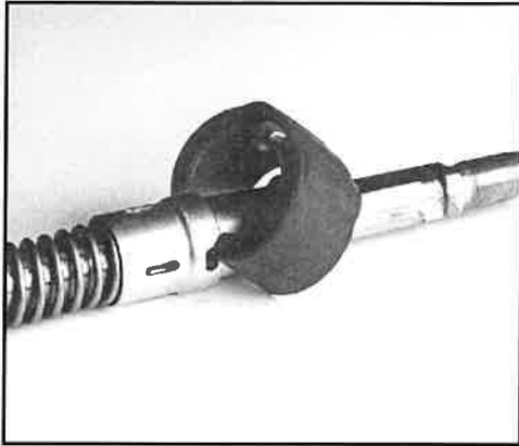
FIG. 41: REMOVE EXHAUST RING
