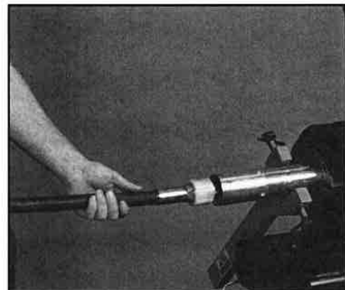
FIG. 40: REMOVE CONTROL STUD
