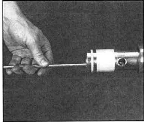
FIG. 71: REMOVE PISTON
